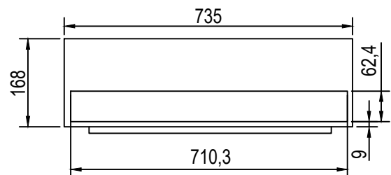
Ausschnitt Maschinenraumblende
