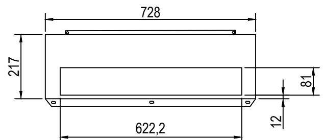
Ausschnitt Maschinenraumblende
